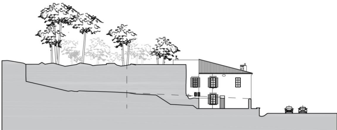
ELEVATION NORD
