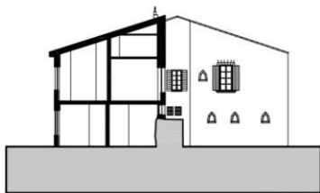
COUPE BB
